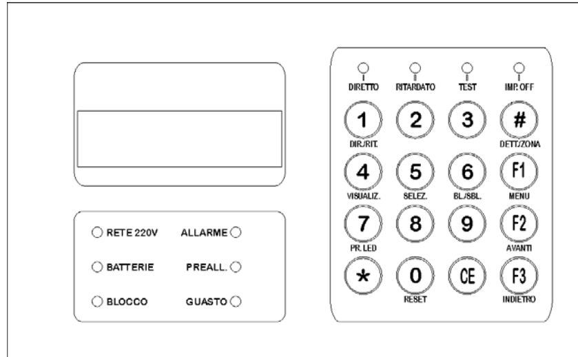
Fig.2: pannello ausiliario
