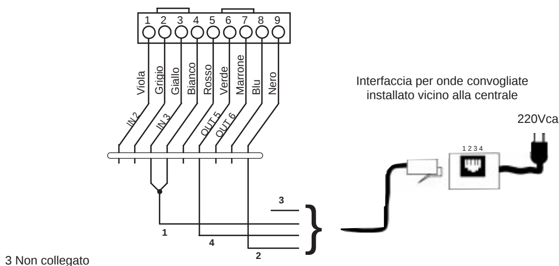
Figura 22. Collegamenti dell'interfaccia per onde convogliate 4300
