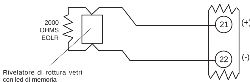
Figura 12. Collegamento dei rivelatori di rottura vetri con memoria alla Zona 8
