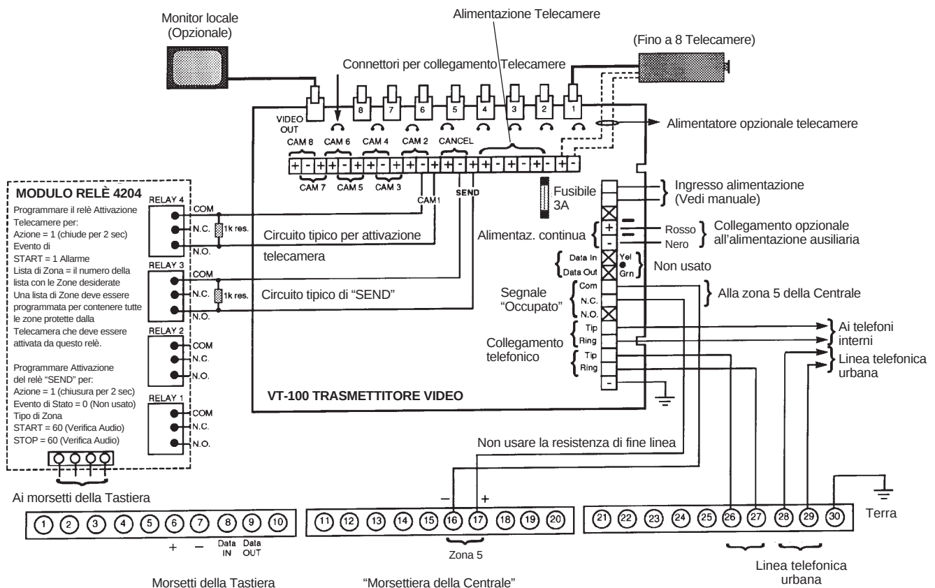
Figura 26. Collegamenti del Modulo di Verifica Video dell'Allarme
