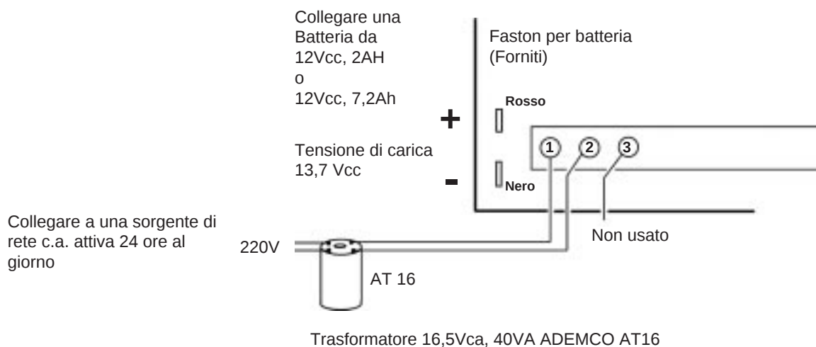
Figura 4. Collegamenti dell'Alimentazione di Rete e della Batteria
